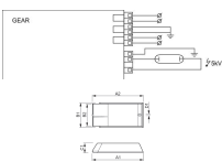
Technische Daten Philips HID-PV C 50 /I CDM 220-240V 50/60Hz für 50W
