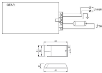
Technische Daten Philips HID-PV C 35 / I CDM 220-240V 50/60Hz für 35W
